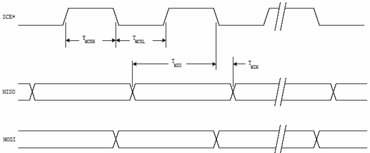
图 7 SPI 主方式时序图 (CKPHA=0)
